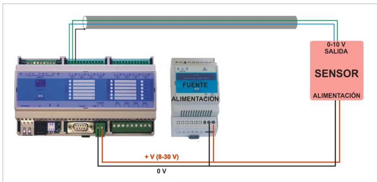
CONEXIÓN DE LAS ENTRADAS ANALÓGICAS
